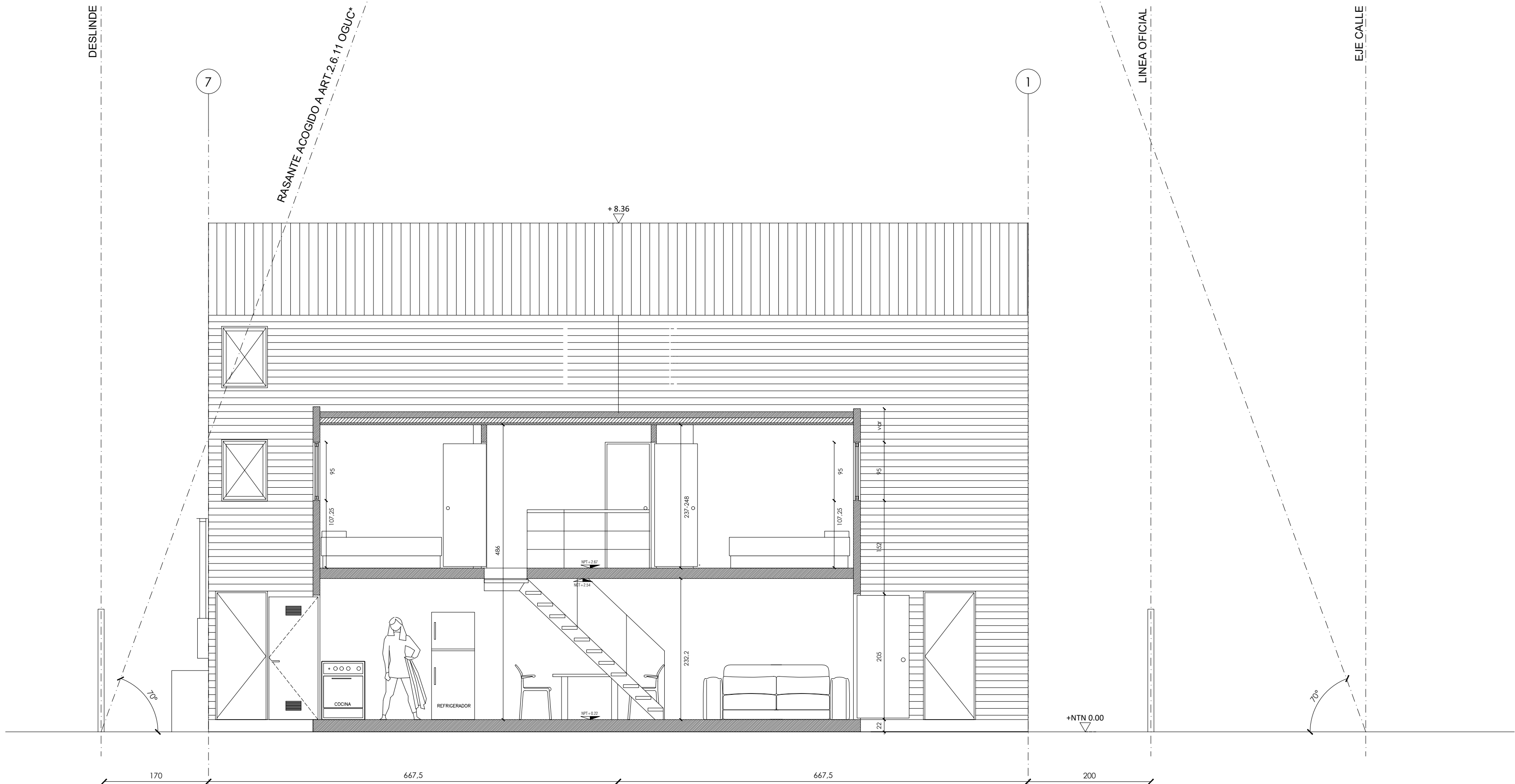
CORTE FF' - ESCALA 1:50
