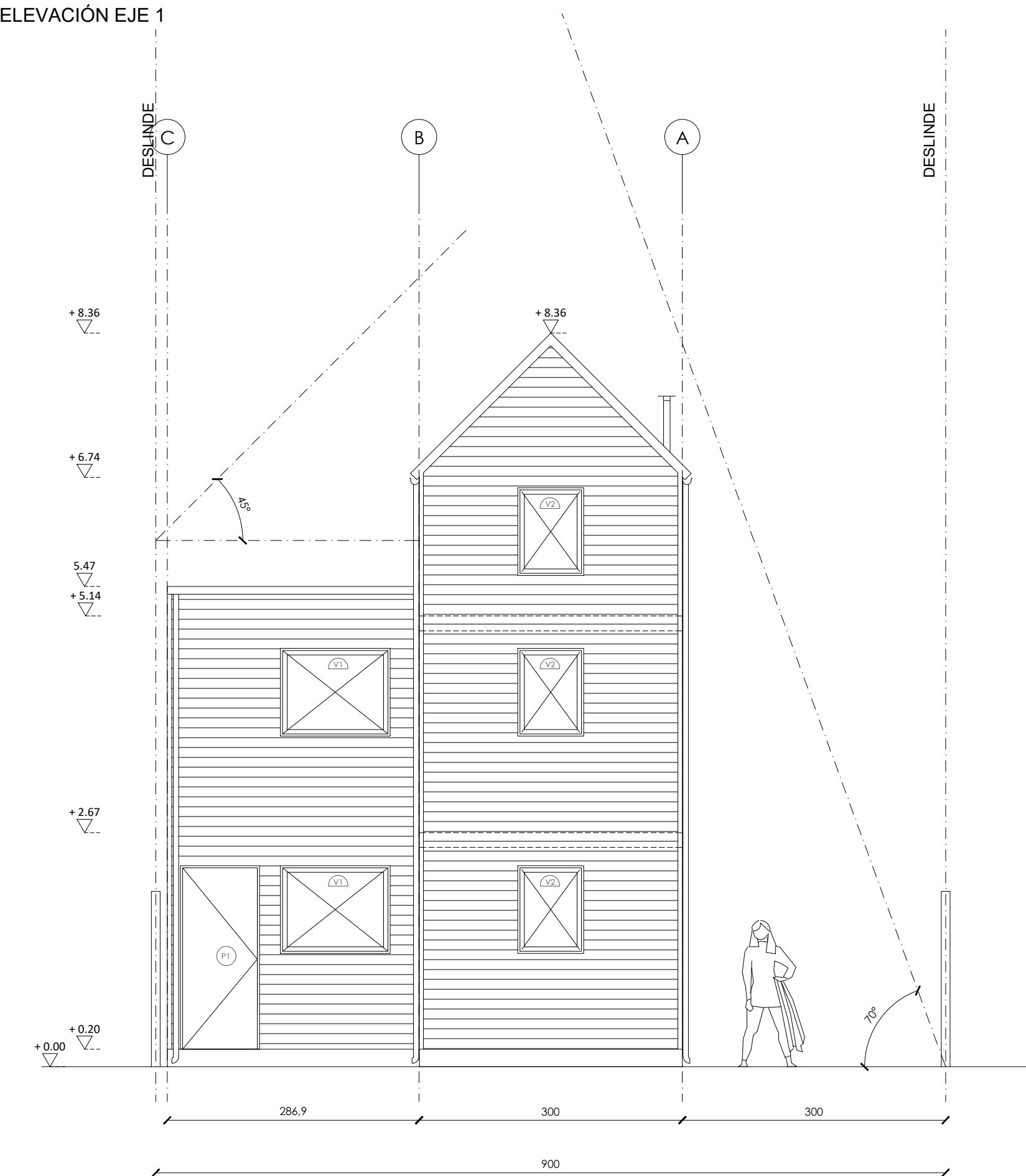
ELEVACIÓN EJE 1
