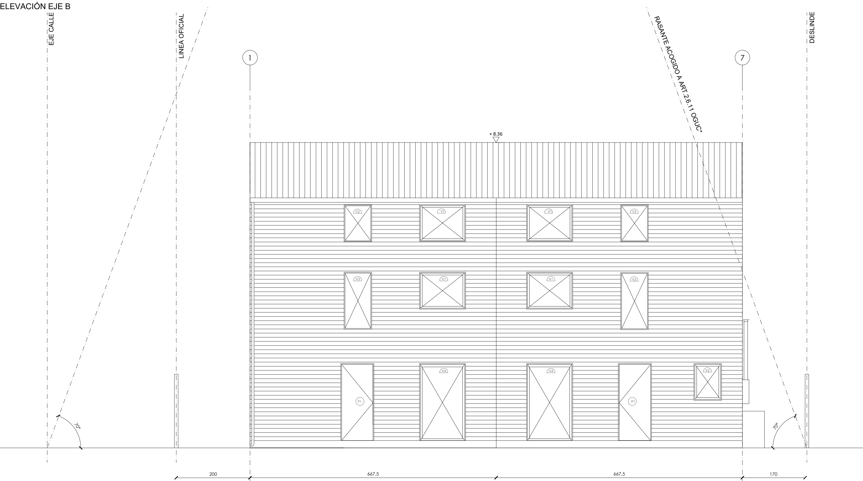
ELEVACIÓN EJE B
