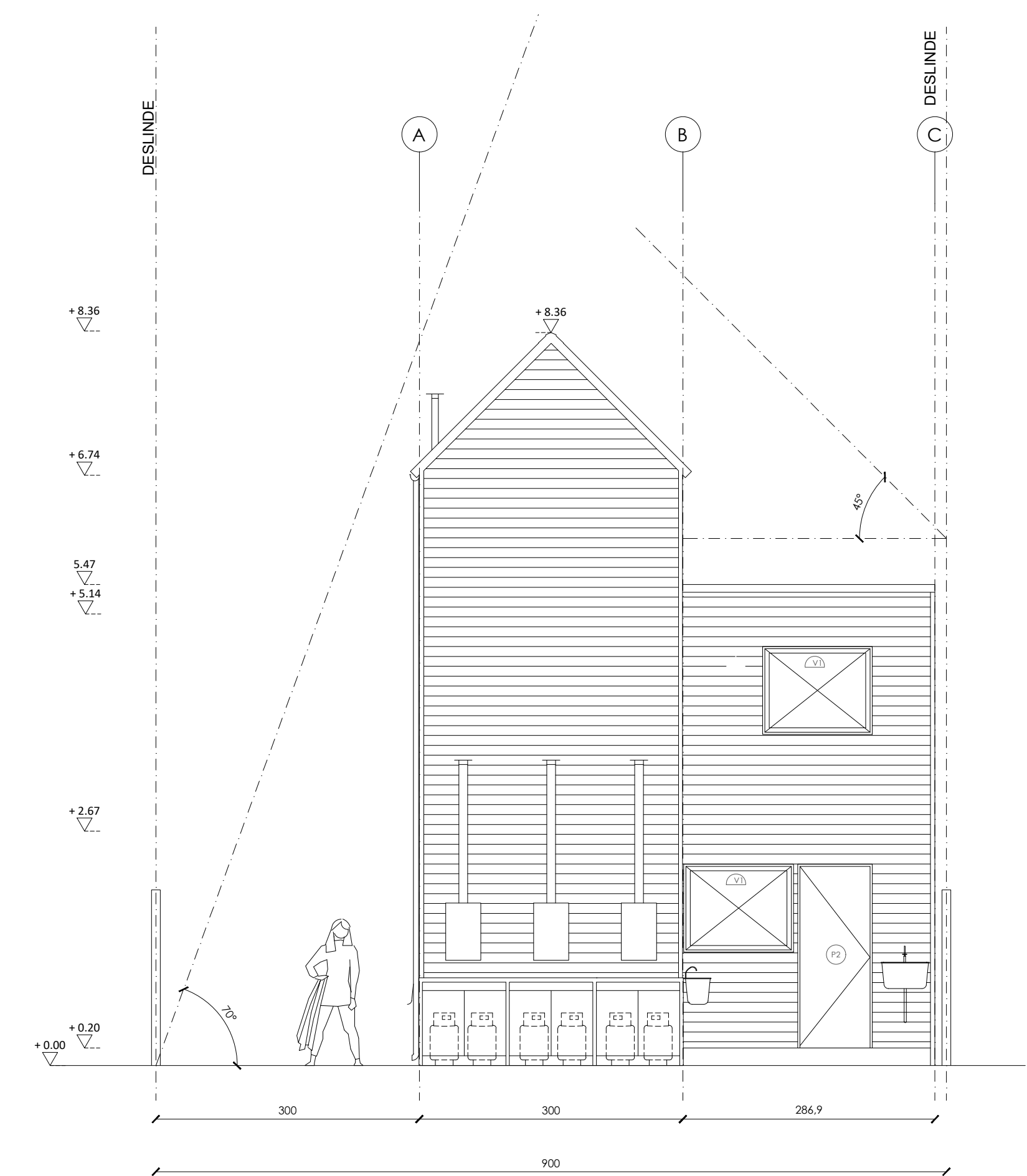
ELEVACIÓN EJE 7
