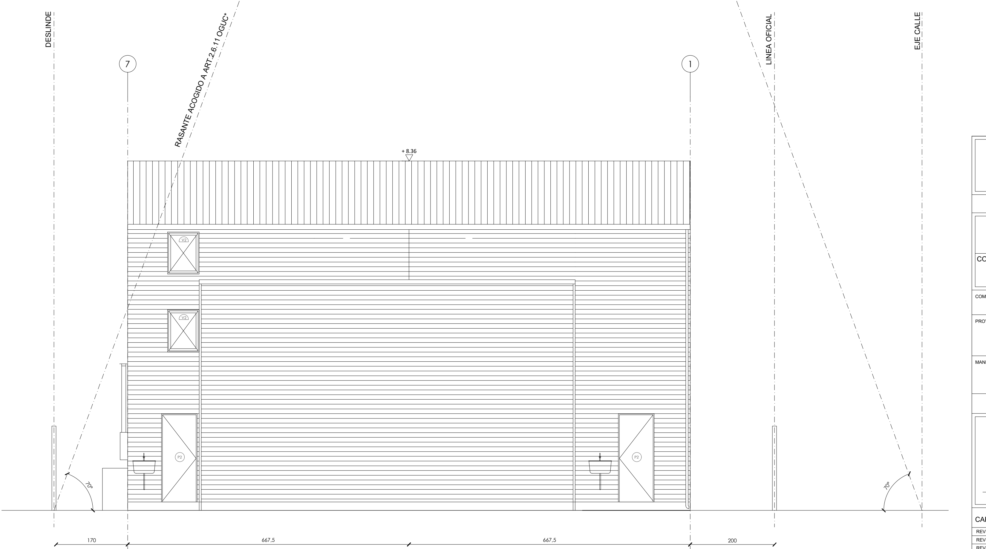
ELEVACIÓN EJE A
