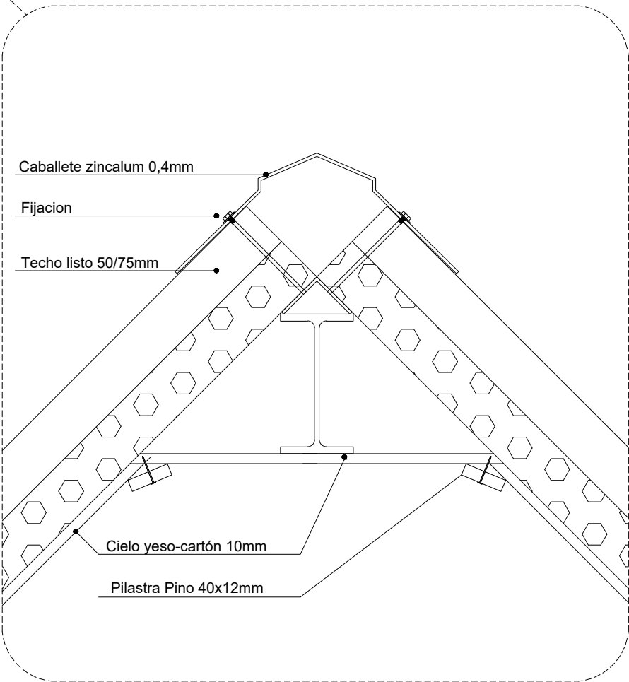
D4 - Techumbre cumbre
