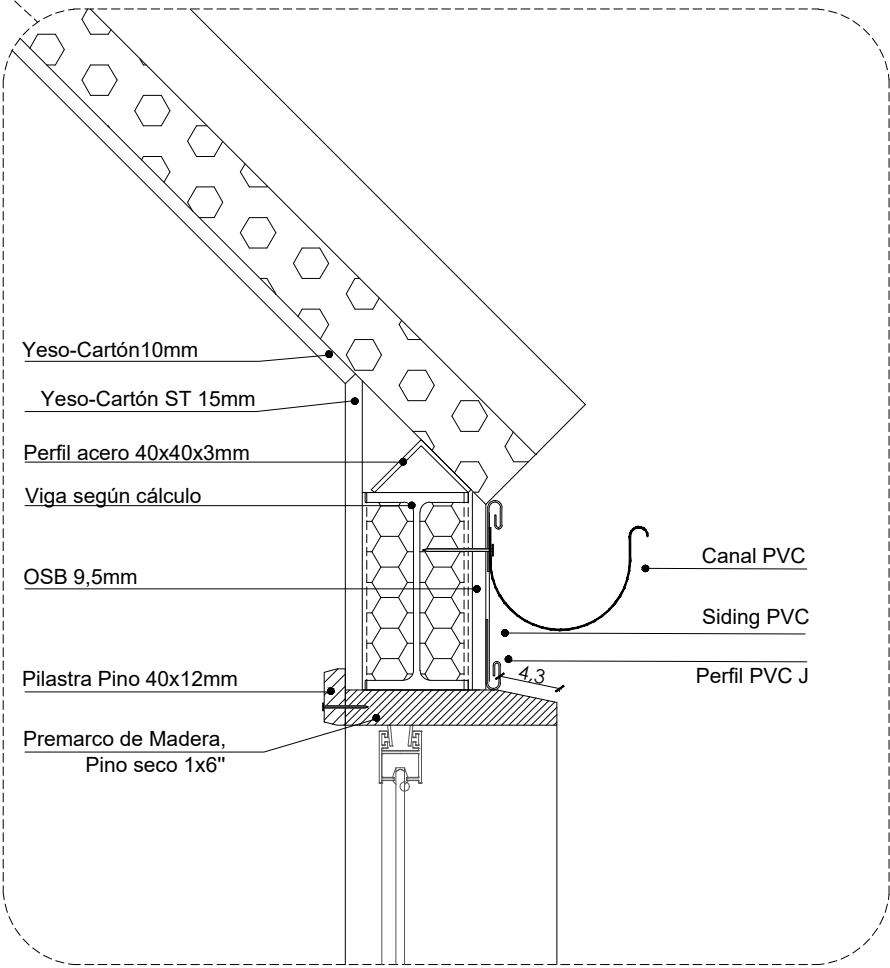
D2 - Techumbre - Cortagotera
